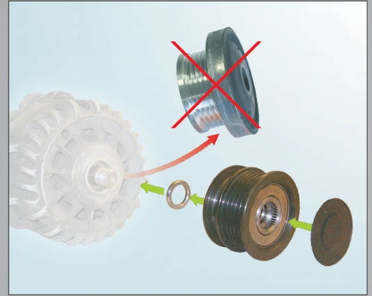
Bild 2: Montageübersicht
